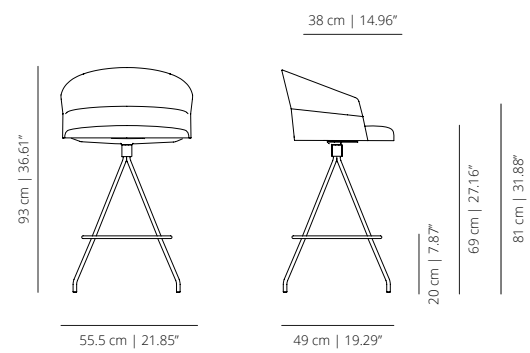
COTGCO stool
